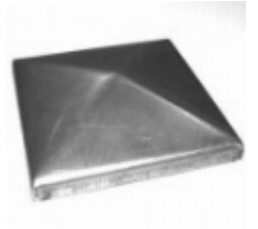
Заглушка на столб 80x80, арт. 15.056.36 80x80x1мм Вес: 0.08 кг Цена: 25 руб.
